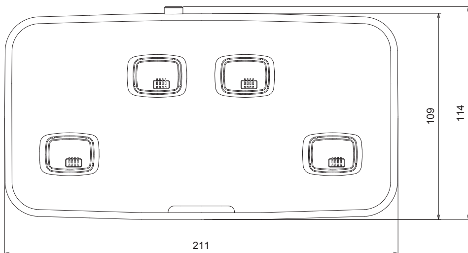
上面図
