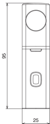
正面図
