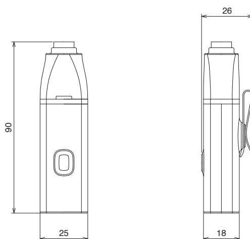
正面図
