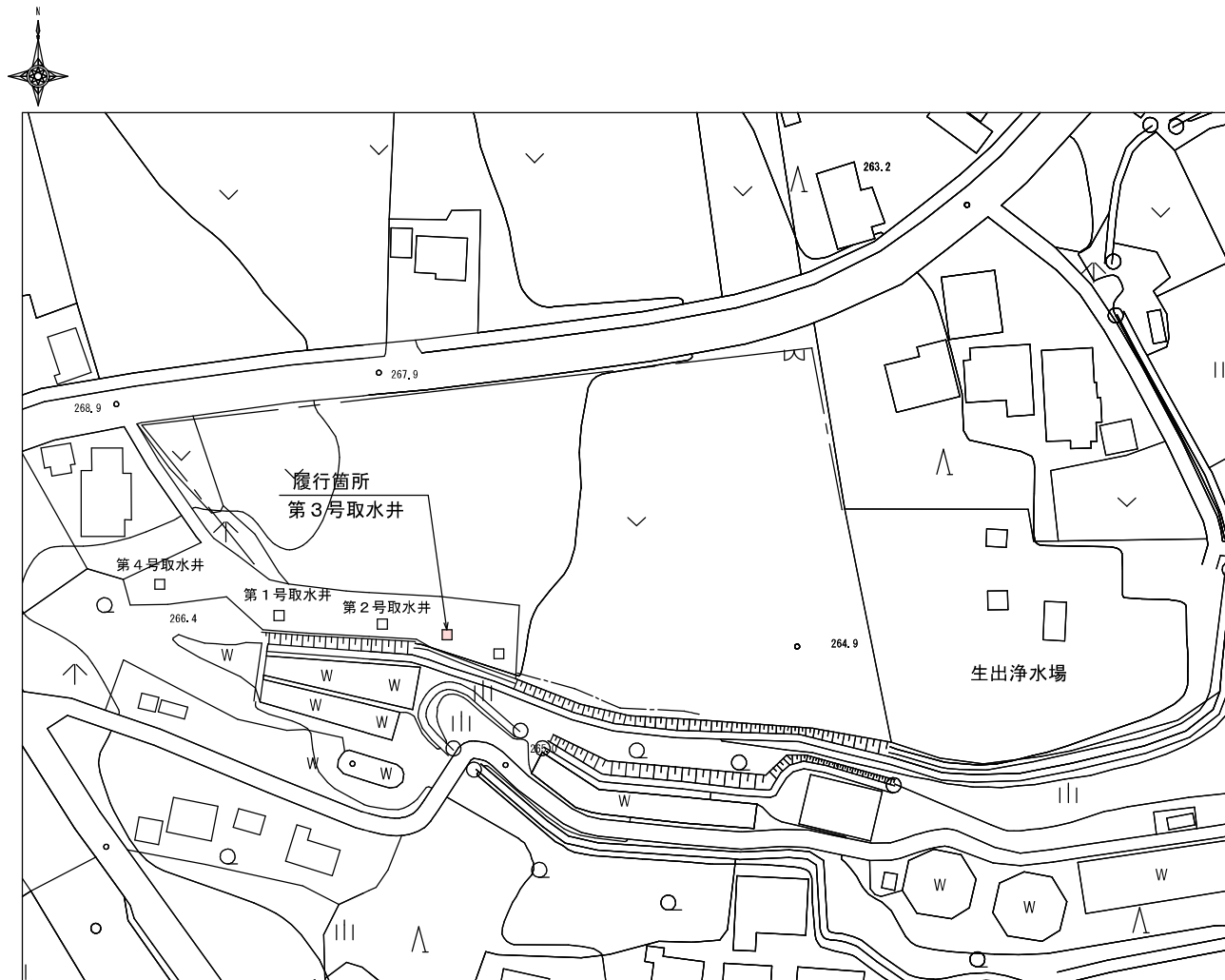
平面図 S=1:500 (生出浄水場)
