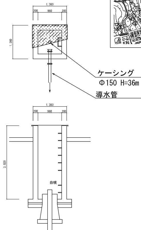
第3号取水井構造図 S=1:30
