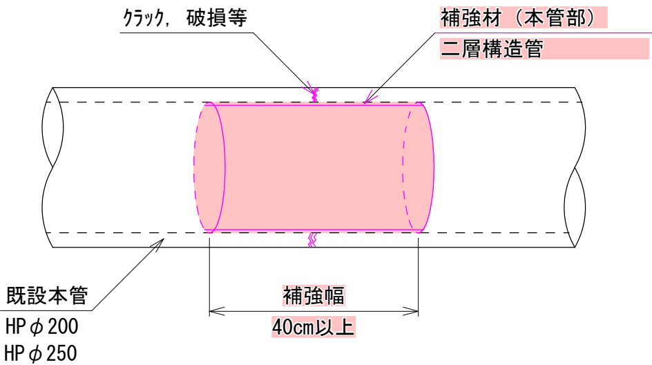
横断面図
