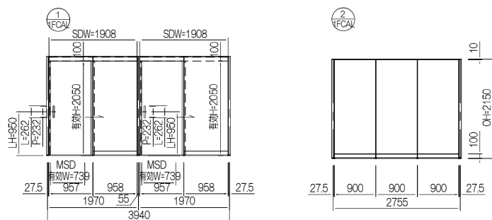
展開図
