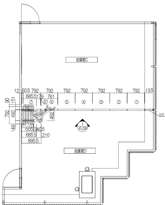
平面図
