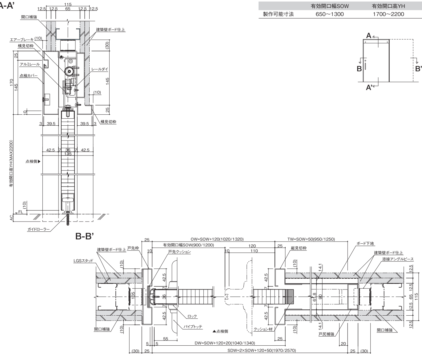
詳細図
