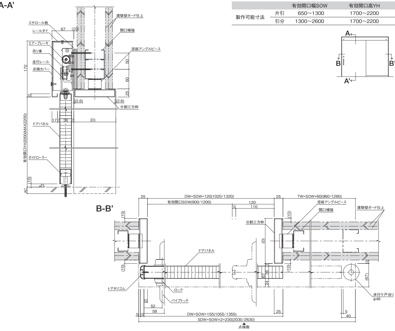
詳細図
