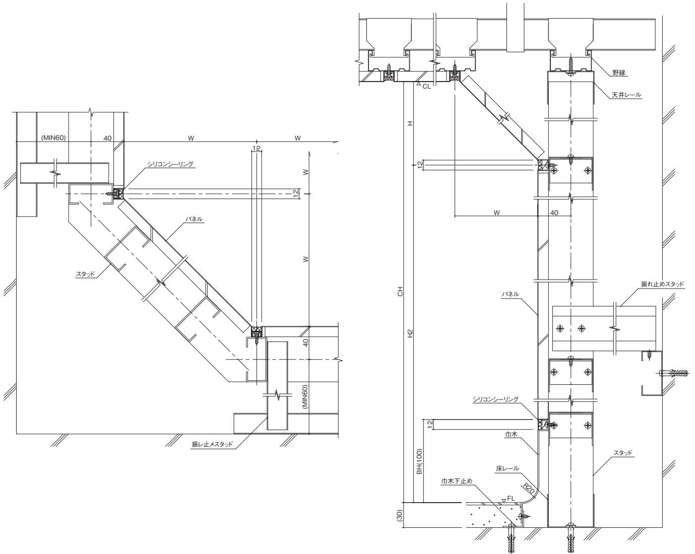
詳細図
