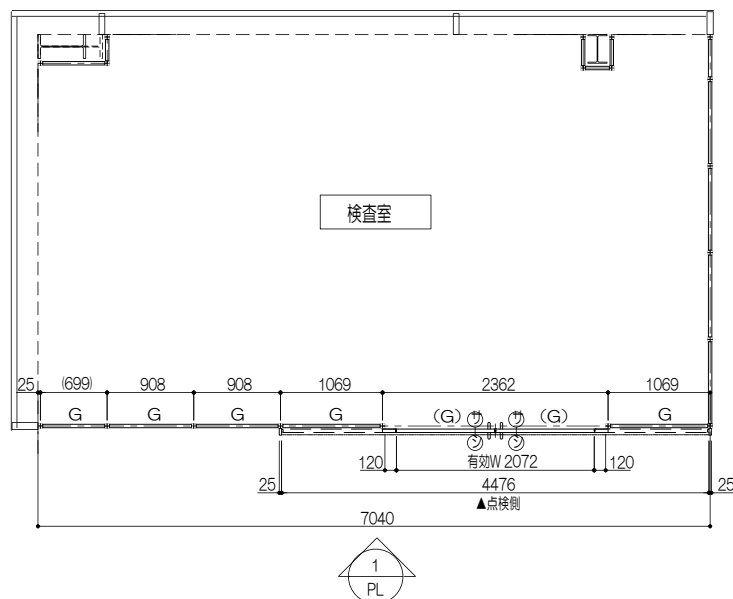
平面図
