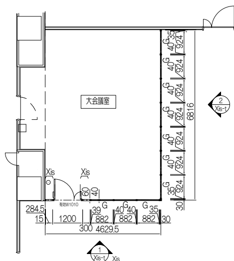
平面図
