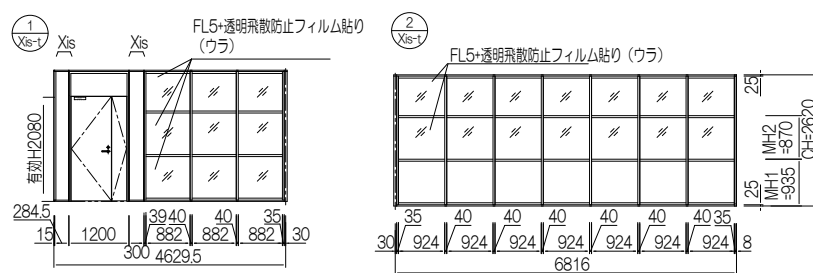
展開図
