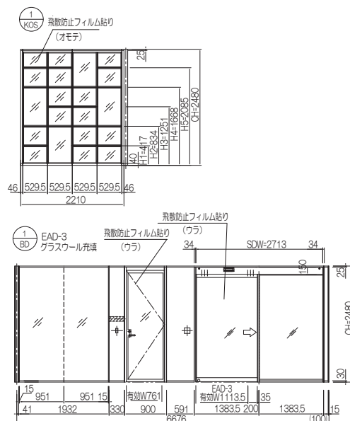
展開図
