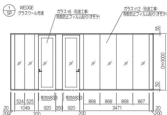
展開図
