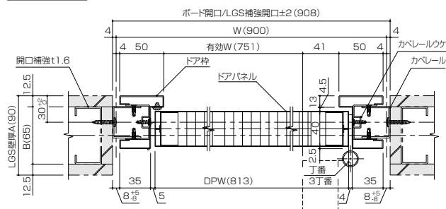
横断面図
