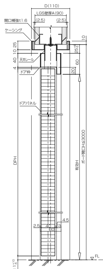
縦断面図
