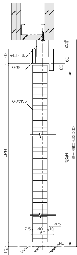
縦断面図
