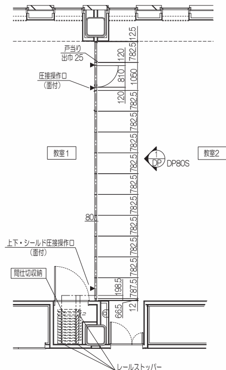
平面図
