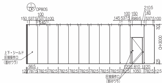
展開図
