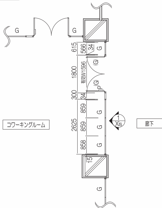
平面図
