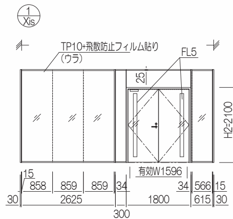
展開図
