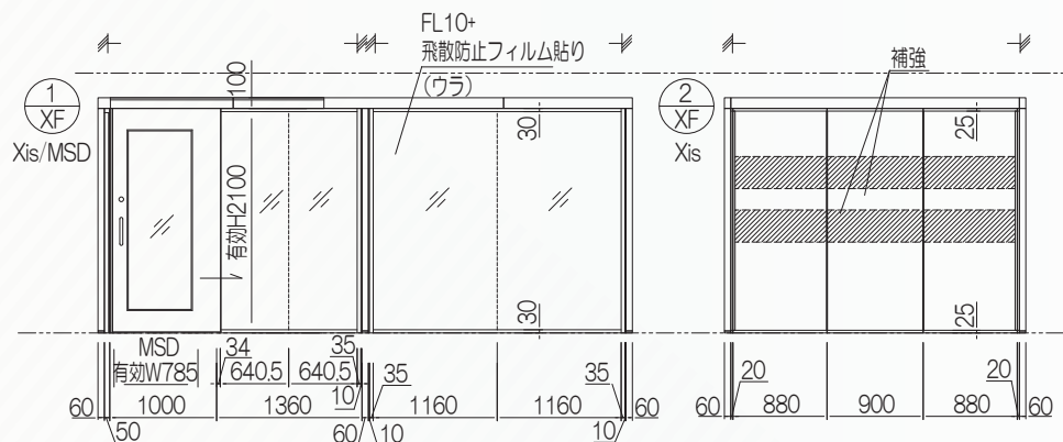
展開図
