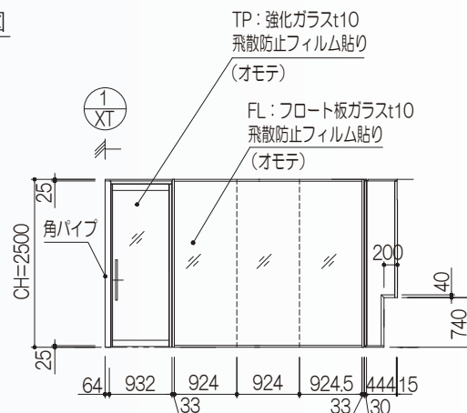
展開図
