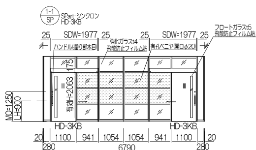
展開図
