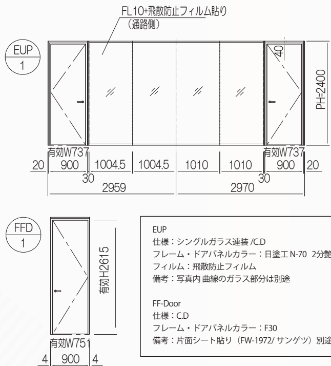
展開図
