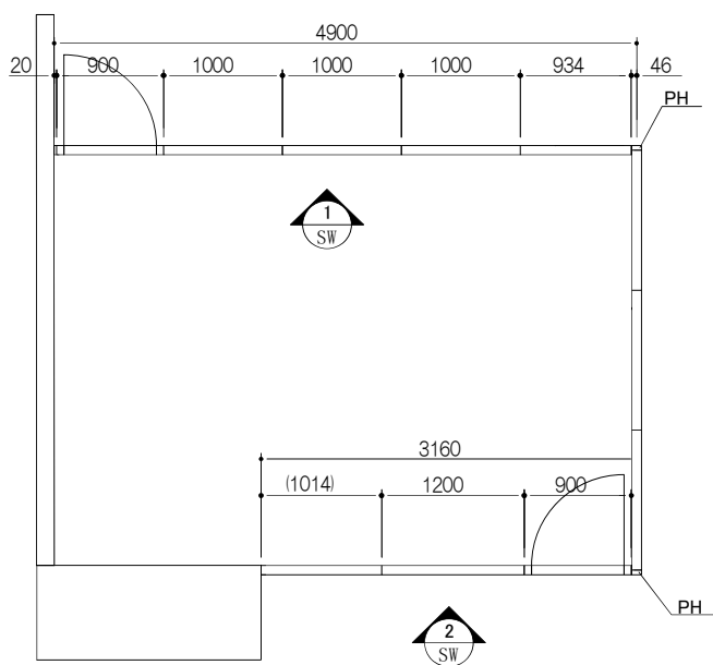
平面図
