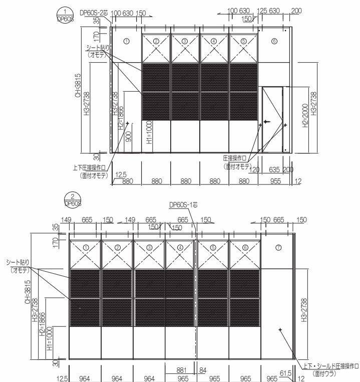
展開図
