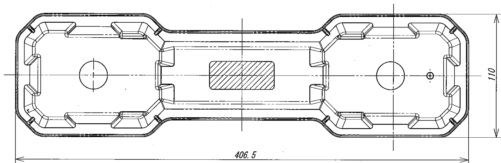
上面図
