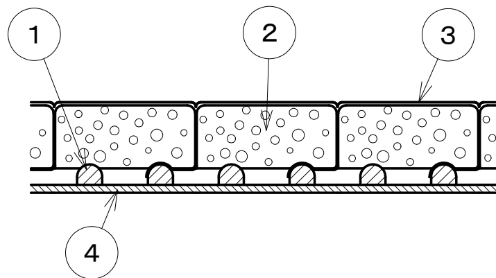
A部 詳細 3／1
