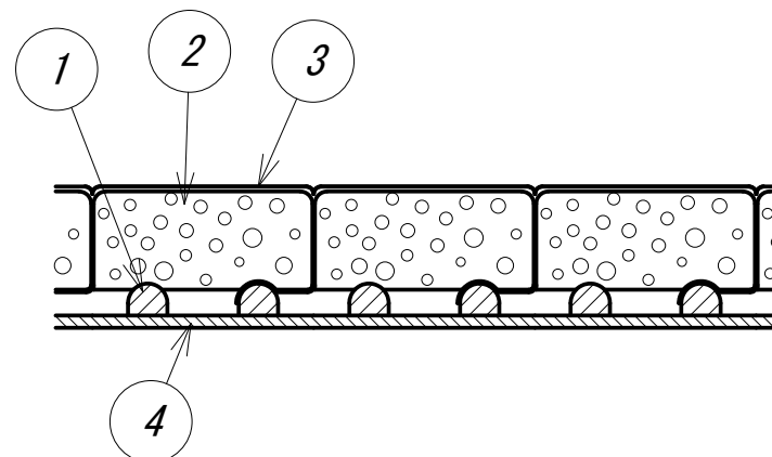
A部 詳細 3／1
