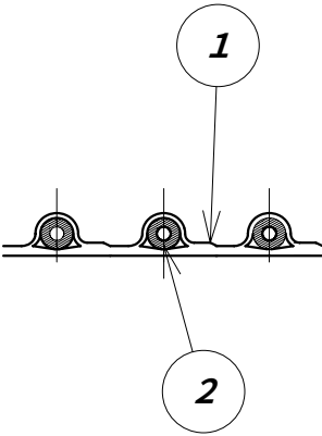
A部詳細図
