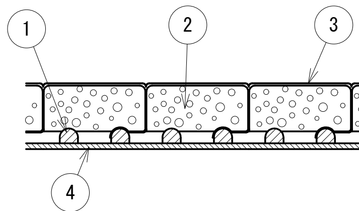
A部 詳細 3 / 1
