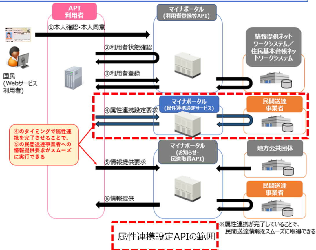
図 2.1-1 属性連携設定 API の概要
