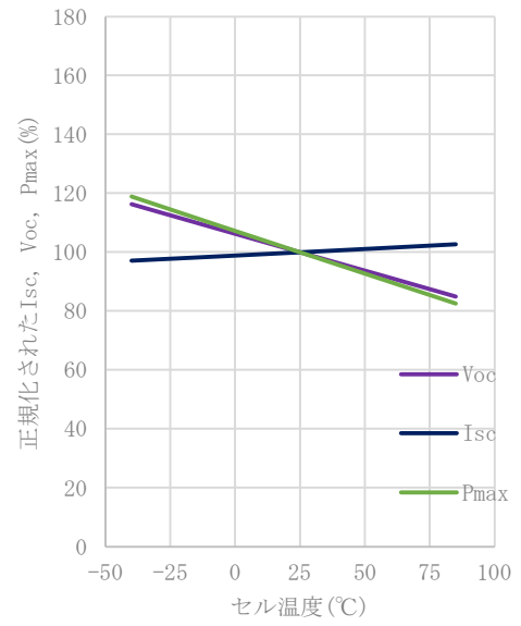
Isc, Voc, Pmax温度依存性
