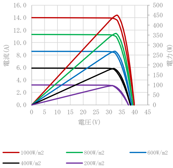
電流-電圧 & 電力-電圧曲線
